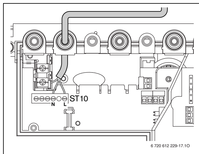
Sl. 25 Spončna letev napajanje ST10
