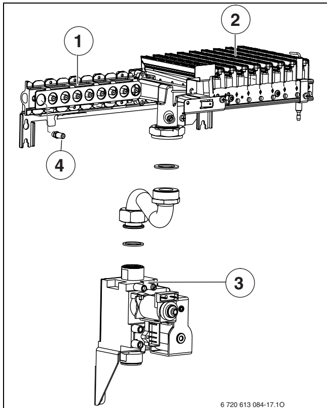
Sl. 55 ZWC 24/28..., ZSC 24/28...
