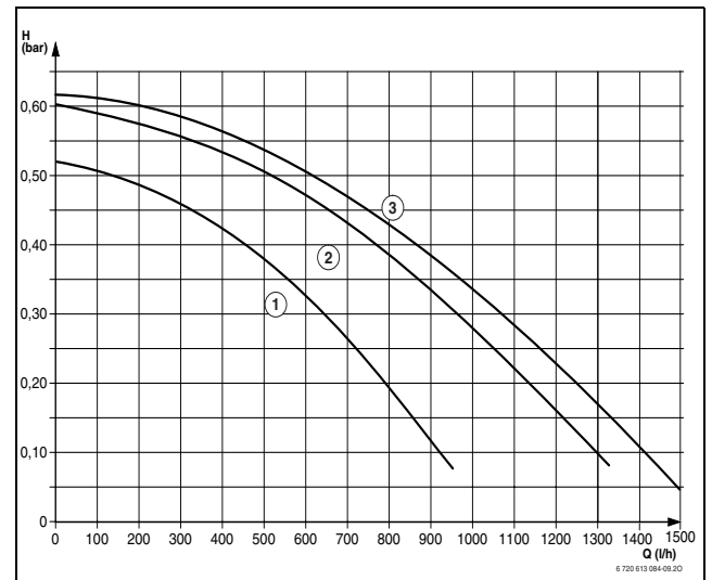
Sl. 39 Karakteristike črpalke pri ZWC 35-3, ZSC 35-3, (brez montažne priključne plošče)
