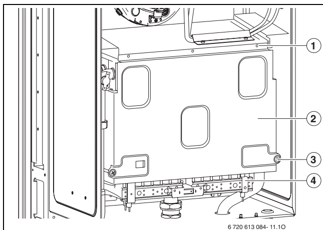
Sl. 54 Odpiranje gorilnika
