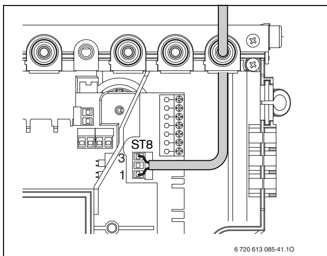
Sl. 23 Prikluček termostata hranilnika
