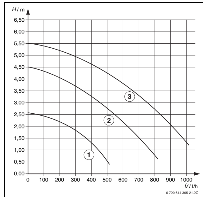
Sl. 40 Karakteristike črpalke (pri obratovanju brez montažne plošče)
