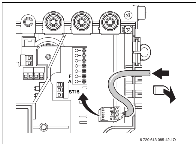
Sl. 22 priključek temperaturnega tipala hranilnika (NTC)
